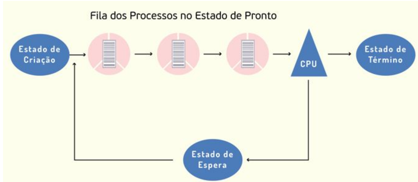
Figura 3 – Escalonamento FIFO
